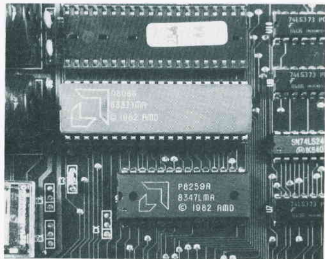
Fig. 2-6. The 8088 CPU.
